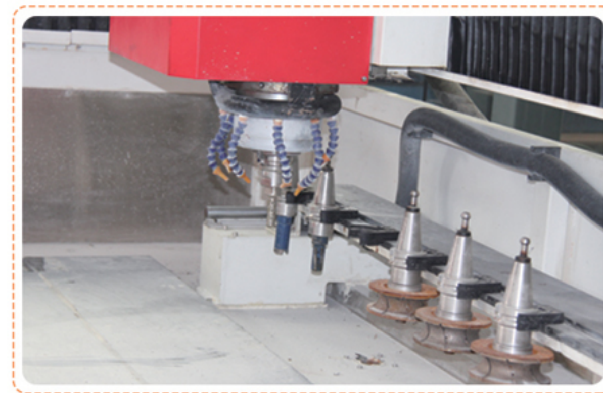
HLCNC3015机型 12个换刀位置
